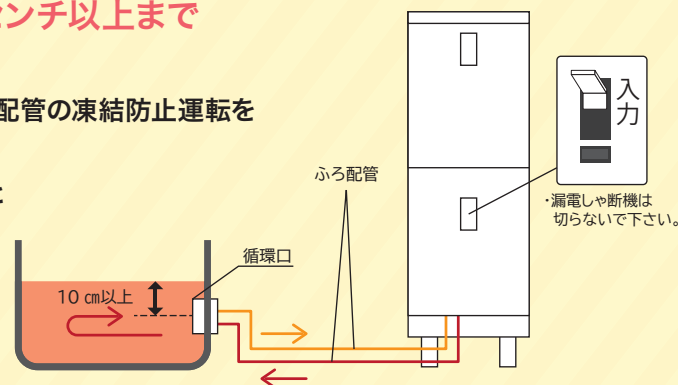
給湯器解説図
